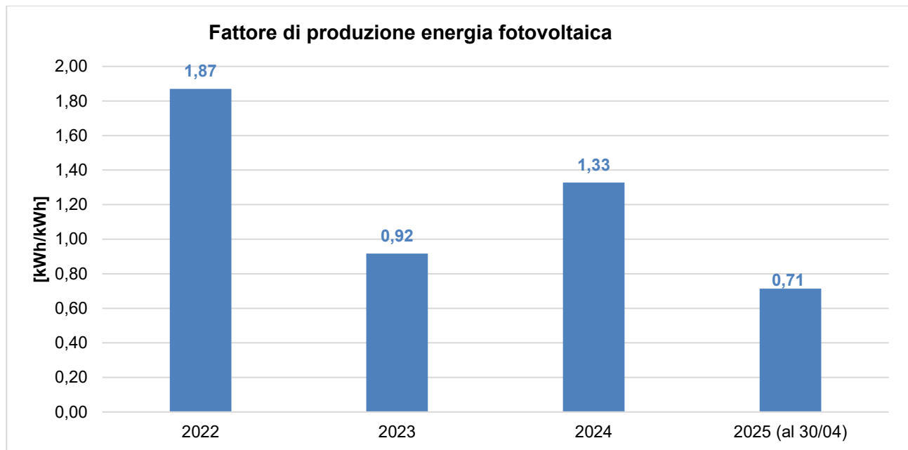
Grafico 4: Andamento del fattore di produzione di energia fotovoltaica nel periodo 2022-2025.
